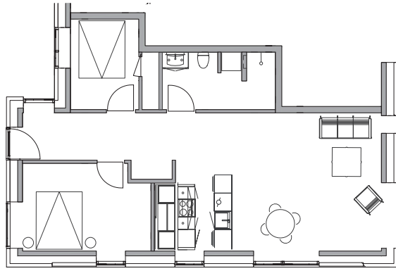
LEJLIGHED TYPE A 87 M 2
