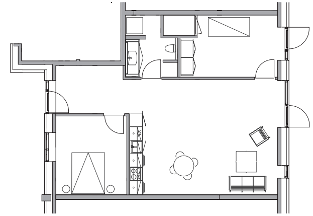
LEJLIGHED TYPE C 89 M 2
