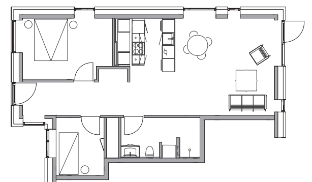
LEJLIGHED TYPE I 86 M 2
