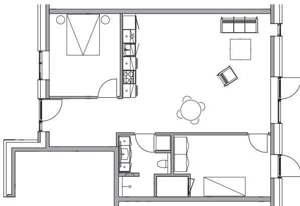
LEJLIGHED TYPE G 92 M 2
